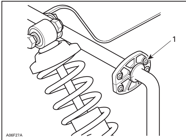
1. Rivets (4)
