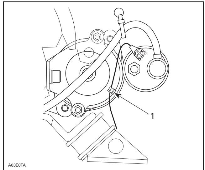
1. Clip
