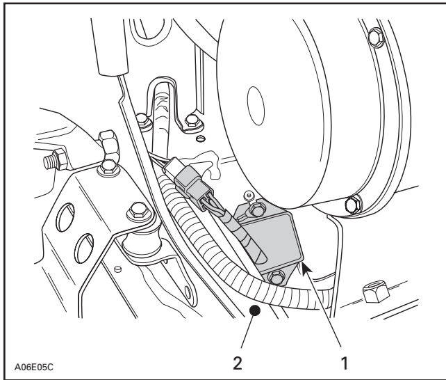
1. Regulator / Rectifier
